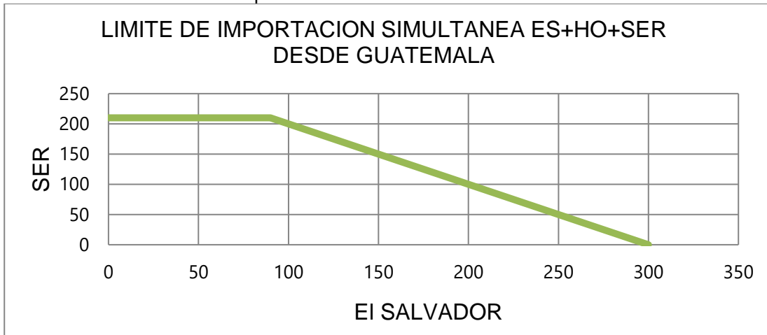
Gráfica 4. Restricción importación de El Salvador + Porteo – demanda máxima
