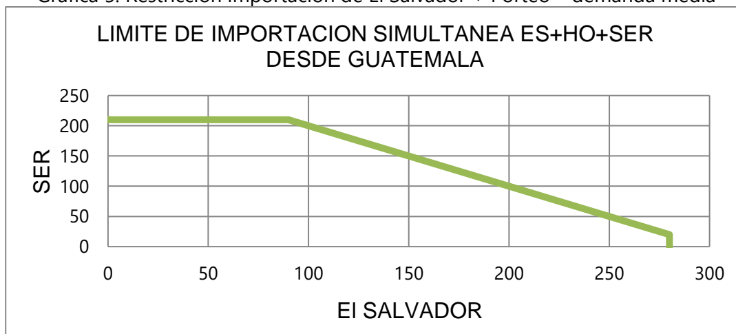
Gráfica 5. Restricción importación de El Salvador + Porteo – demanda media
