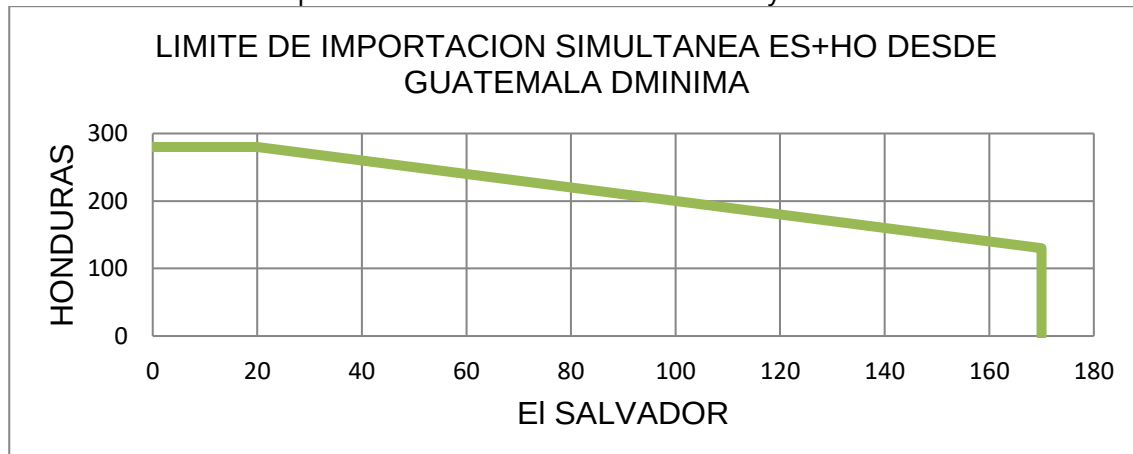
Gráfica 3. Restricción importación simultánea de El Salvador y Honduras– demanda mínima
