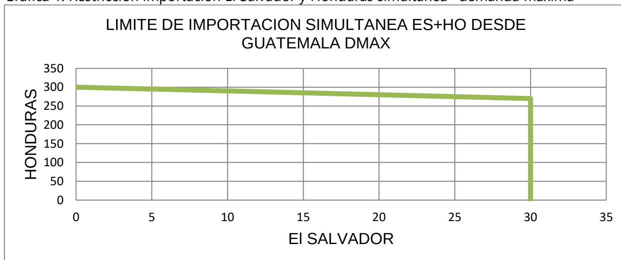
Gráfica 1. Restricción importación El Salvador y Honduras simultánea– demanda máxima
