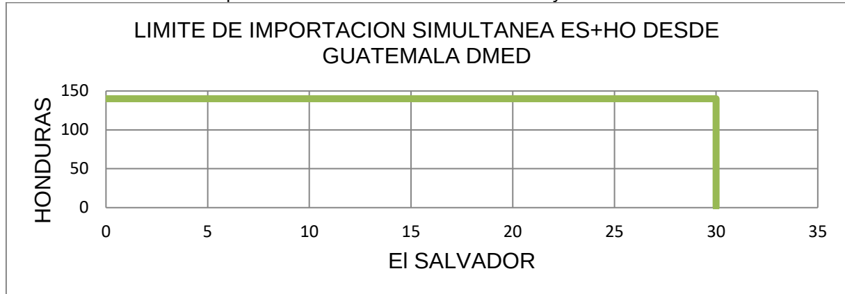
Gráfica 2. Restricción, importación simultánea de El Salvador y Honduras– demanda media.
